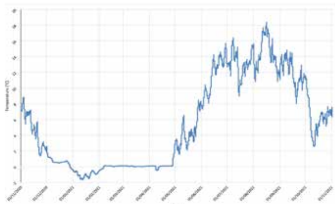
Fig.14 - Grafico andamento temperatura suolo con logger L07
