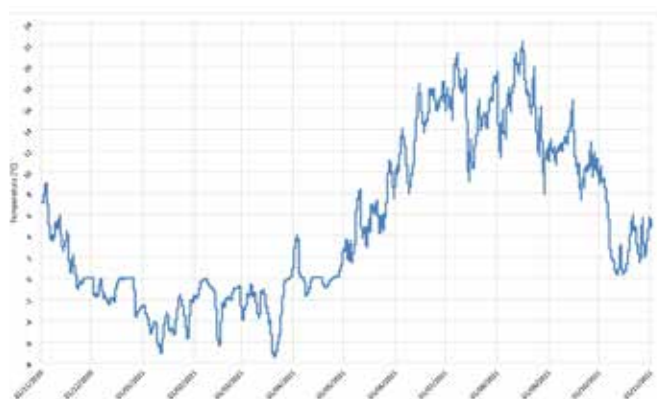
Fig.16 - Grafico andamento temperatura suolo con logger L09
