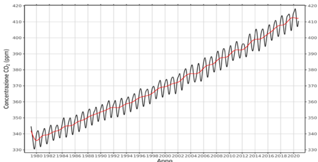
Figura 3 - Serie storica dei dati di concentrazione di CO 2 in atmosfera presso la stazione del C.A.M.M. di Monte Cimone
