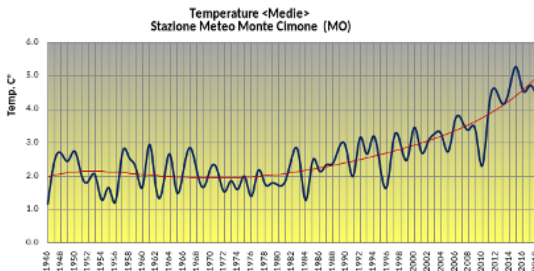
Figura 2 - Temperature medie relative a Monte Cimone (cortesia C.A.M.M. Centro Aeronautica Militare di Montagna)
