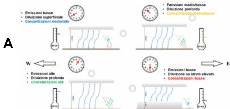
Figura 3 - A - Evoluzione diurna della concentrazione dei composti organici volatili biogenici (BVOC) nelle giornate calde e serene, adattato da [56]
